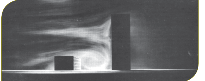
منوع شدن برجهای در مقابل جریان باد. یک ساختمان بلند مرتبه به میزان ده ها ساختمان کوتاه تر وزش مناسب باد در گذرگاه ها و تپه های شهری جلوگیری می کند.
