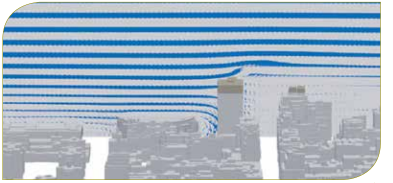
نزول جریان باد در جلوی برجها و کمک به افزایش آلودگی
