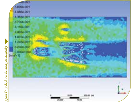
منوع شدن برجهای در مقابل جریان باد. یک ساختمان بلند مرتبه به میزان ده ها ساختمان کوتاه تر وزش مناسب باد در گذرگاه ها و تپه های شهری جلوگیری می کند.
